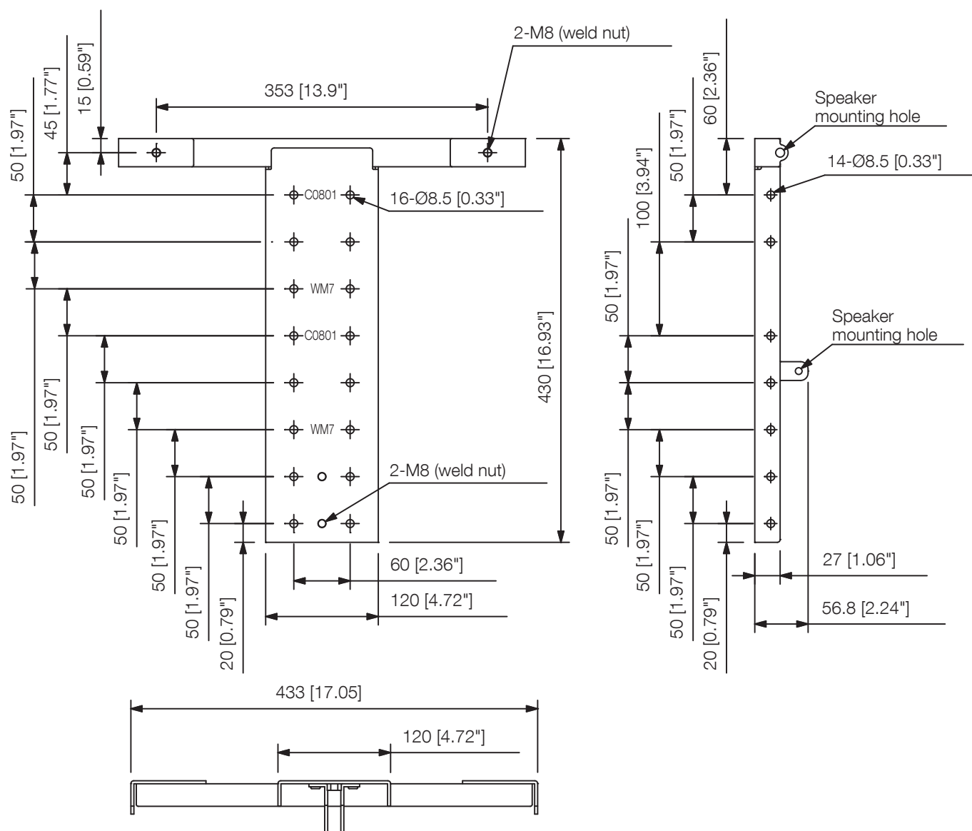
T-bracket
