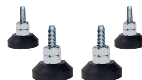
BT856-FEET – regulowane nóżki z funkcją poziomowania do instalacji wolnostojącej (pak. 4szt)
