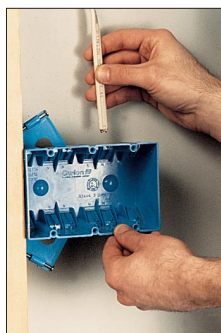
Align Wire
